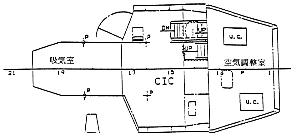
第1甲板
