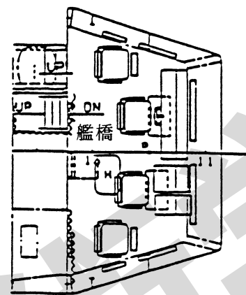
01甲板
